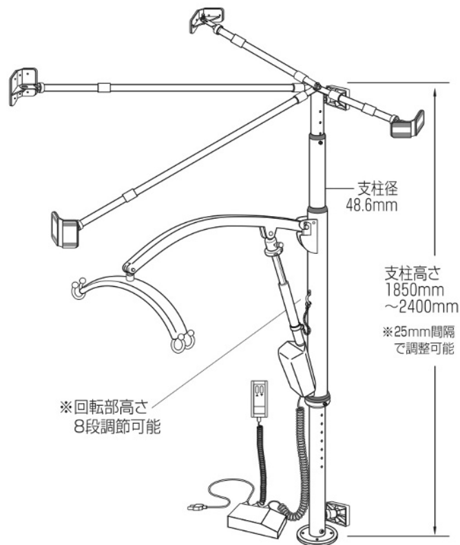
■F1SKKセット外観寸法
