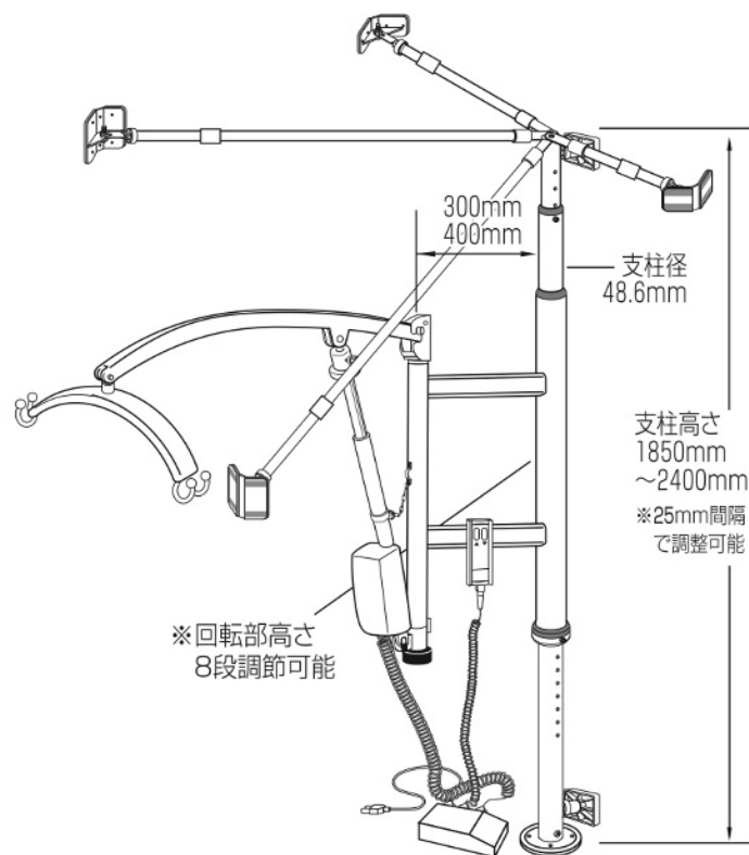
■F2RSKKセット外観寸法
